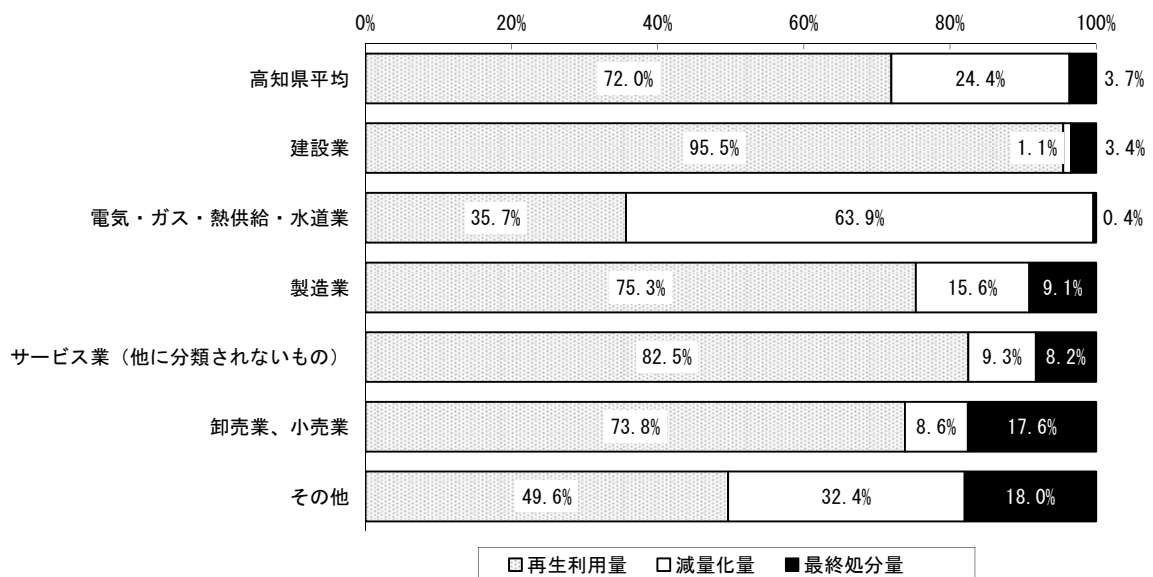
図 3-1-4 業種別の処理・処分状況（令和元年度）
