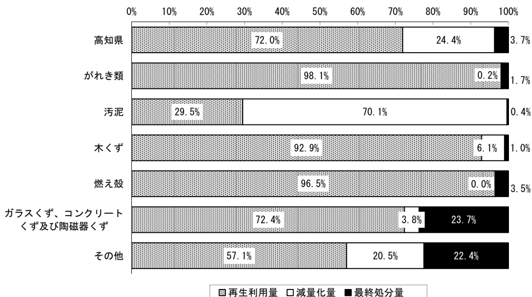
図 3-1-5 種類別の処理・処分状況（令和元年度）
