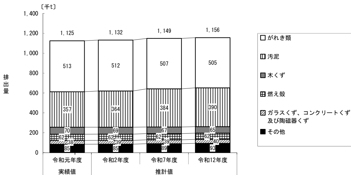
図 3-3-2 排出量の将来推計（業種別・種類別）
