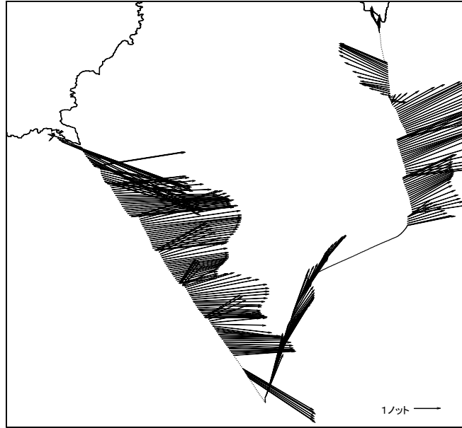
図2 沖合定線における流向・流速
