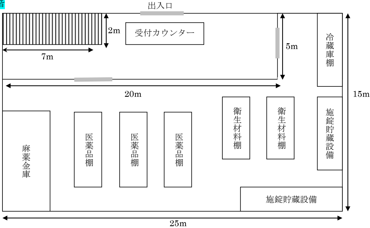
営業所の平面図
