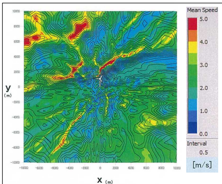
年平均風速分布図（地上高20.6m(ハブ高さ) 50mメッシュ）
