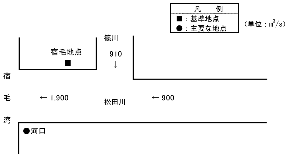
松田川計画高水流量図
