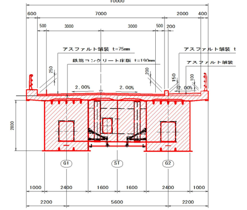
橋梁部 標準断面図
