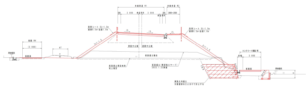
土工部 標準断面図
