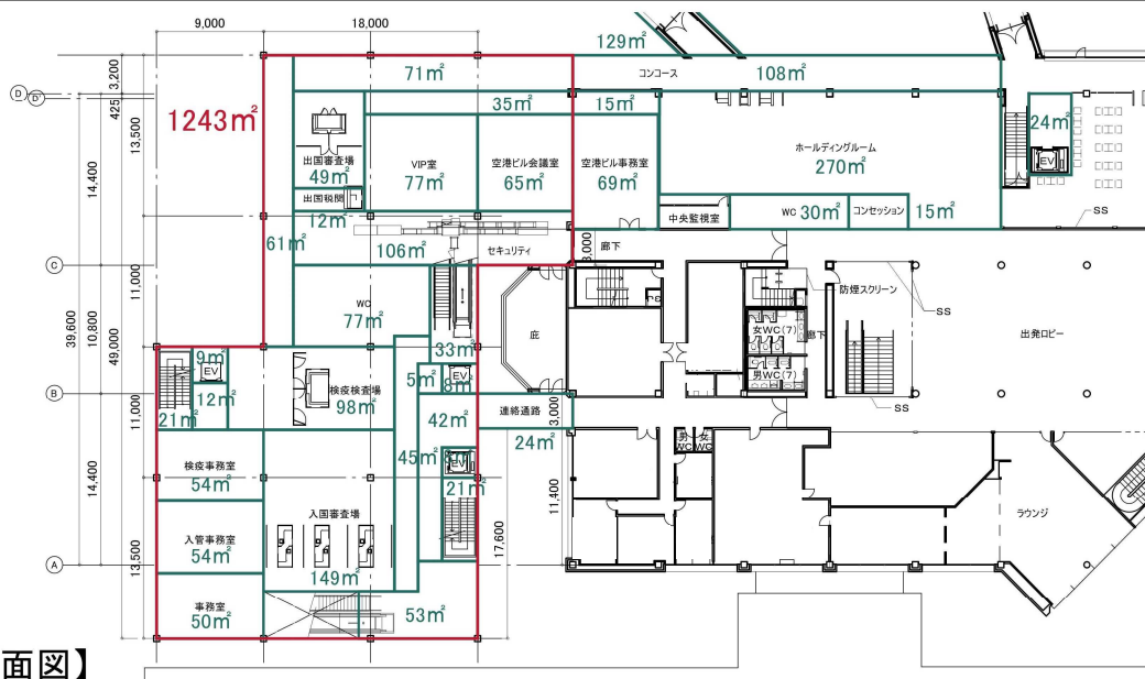
【3階平面図】
