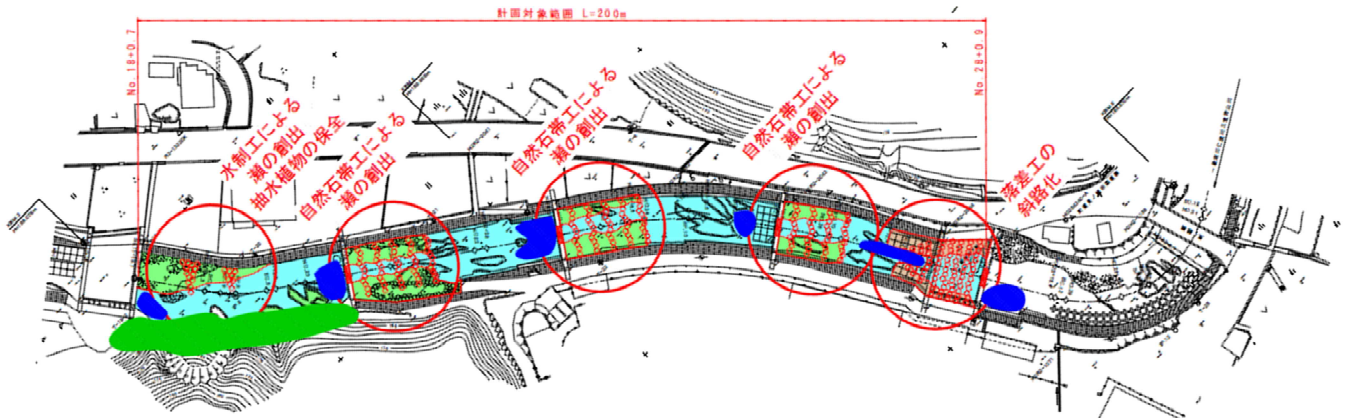
【計画平面図】
