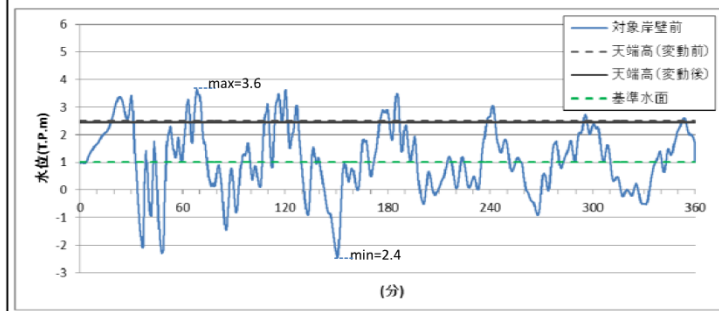
【水位波形】
