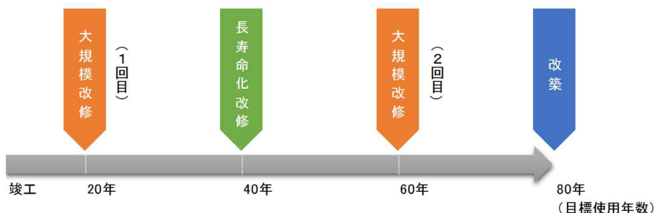
図 6.1 長寿命化の基本的な改修周期
