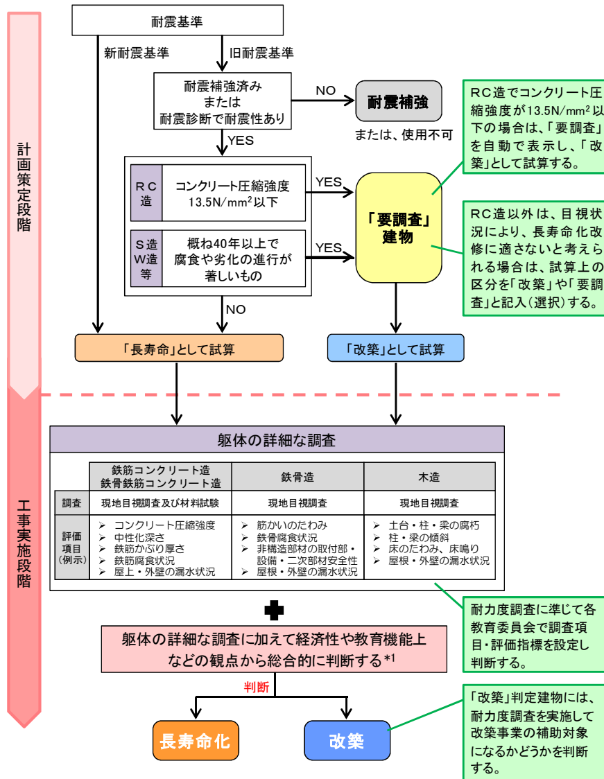
図 3.1 長寿命化の判定フロー（「学校施設の長寿命化計画策定に係る解説書」（文部科学省））
