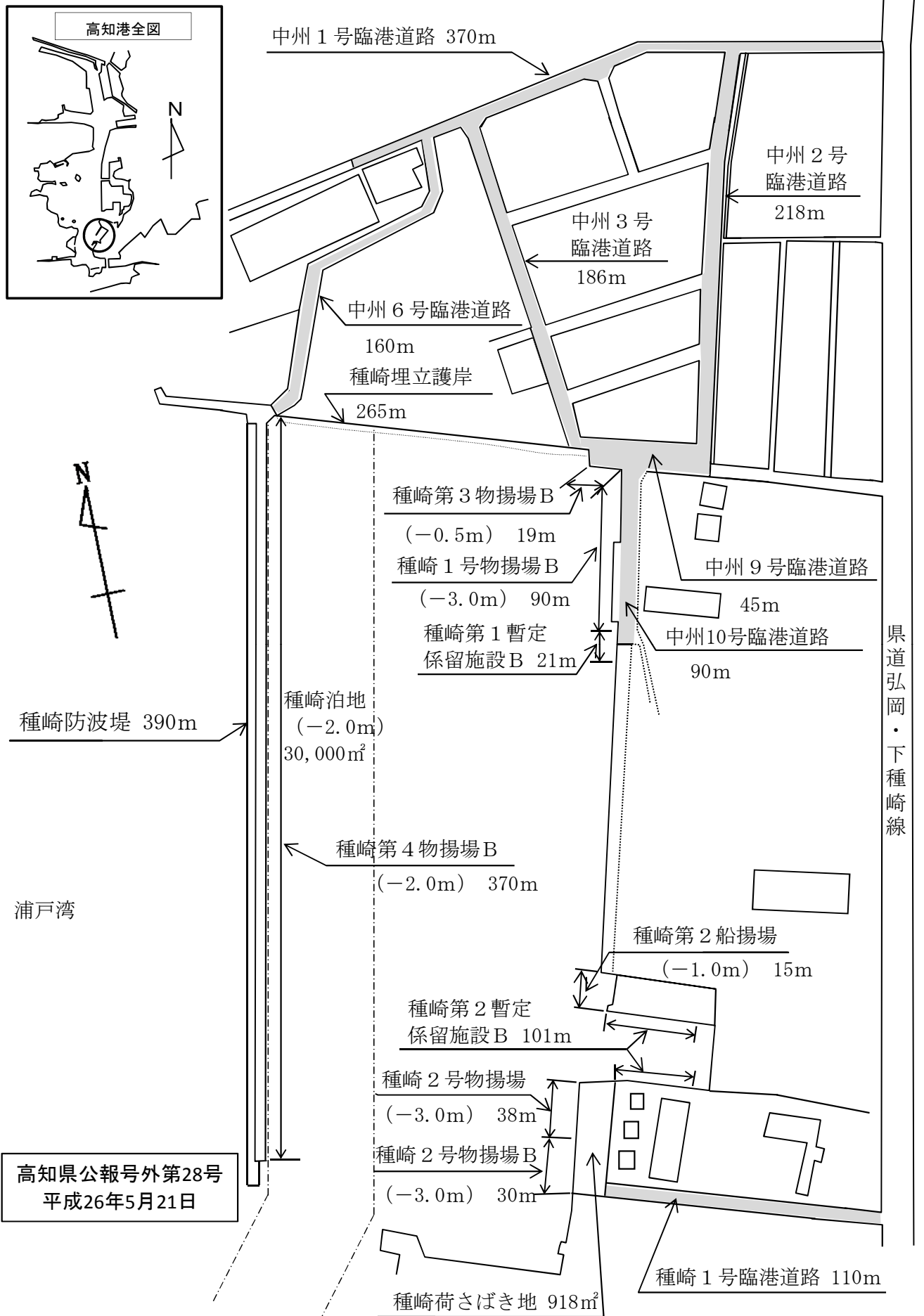
別図8 高知港種崎物揚場等の区域図
