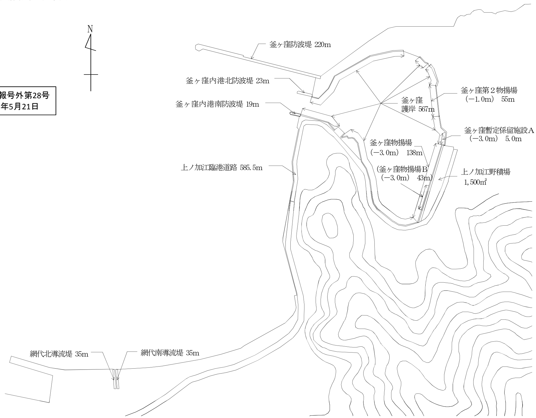
別図39 上ノ加江港物揚場等の区域図
