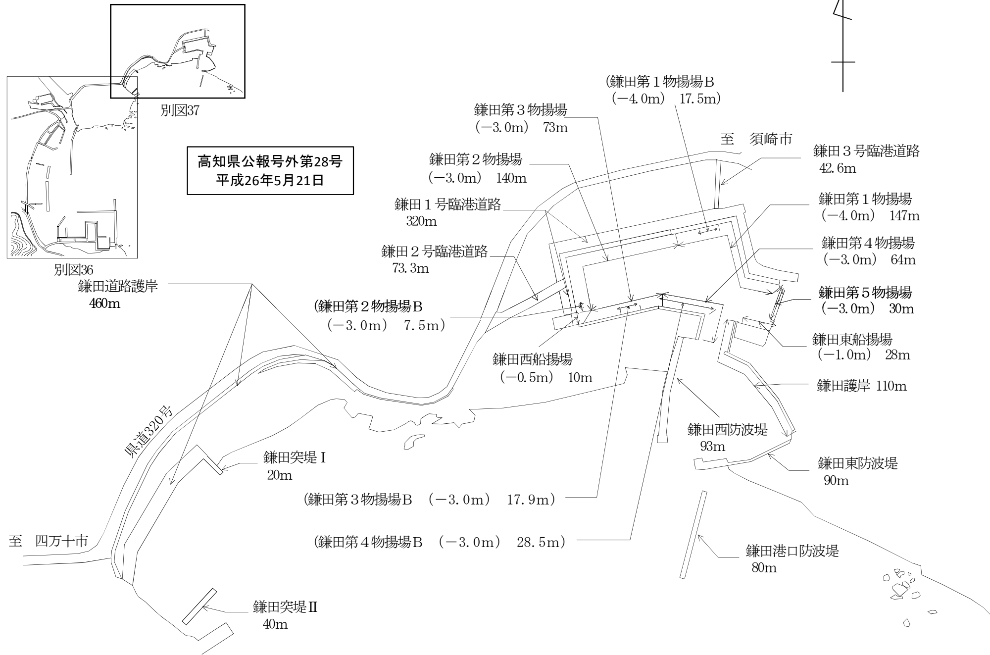
別図37 久礼港鎌田物揚場等の区域図
